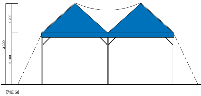
立面図
